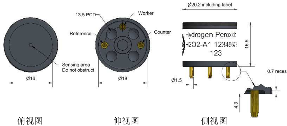
图1 H2O2-A1示意图
