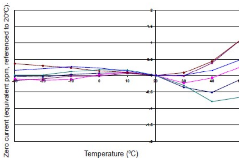
图2 零点温度特性
