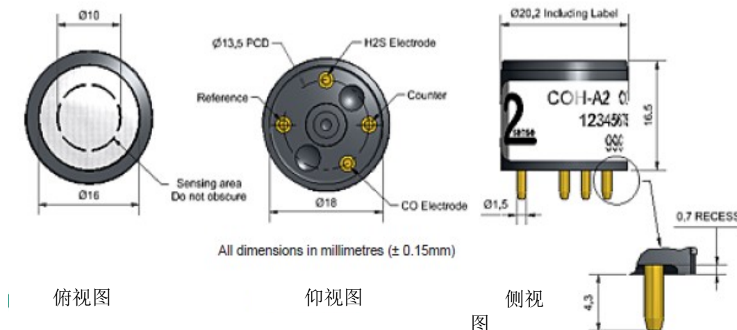
图4 传感器图示
